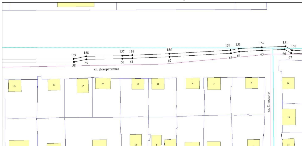
Выносной лист 8
