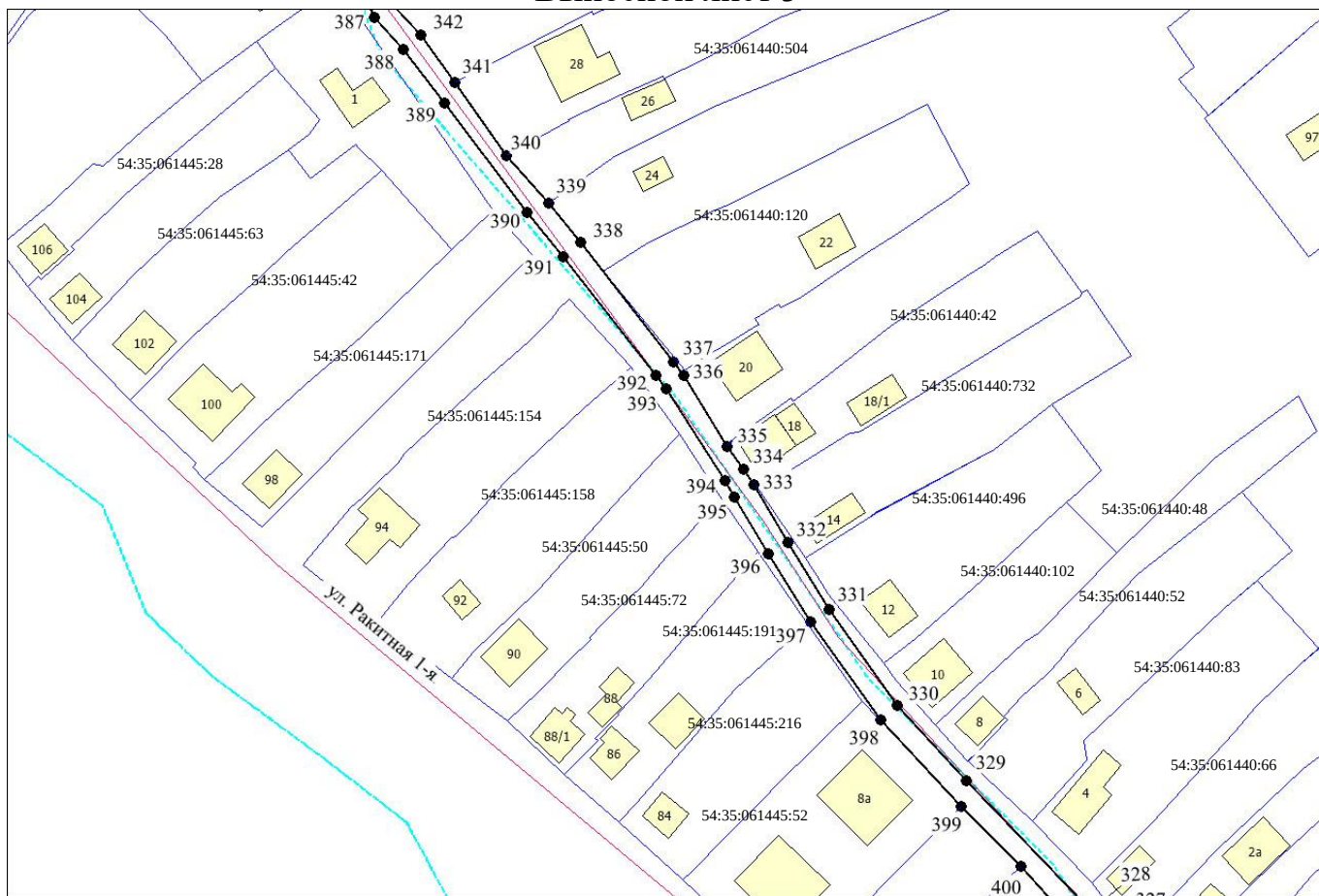
Выносной лист 3
