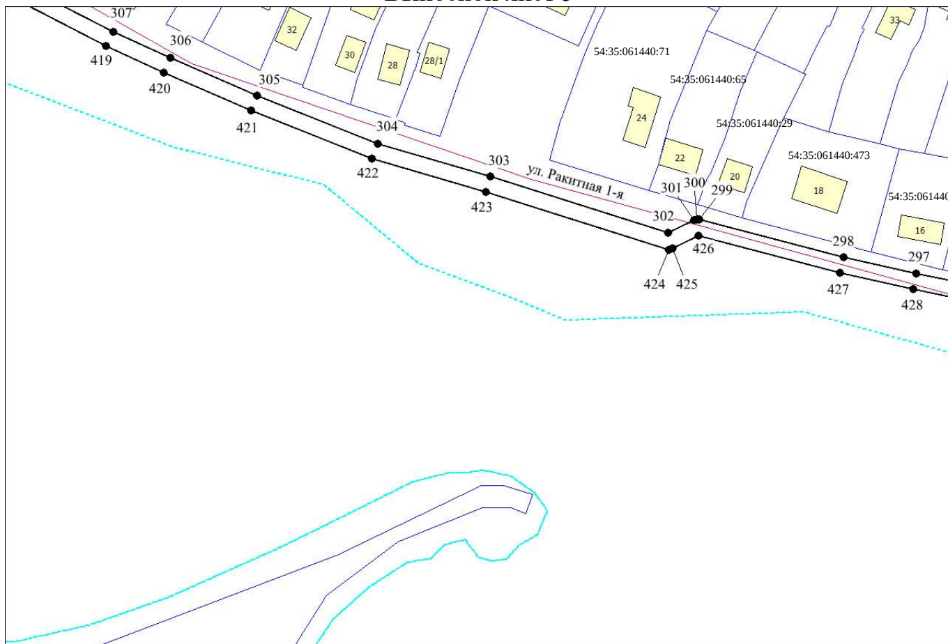
Выносной лист 5
